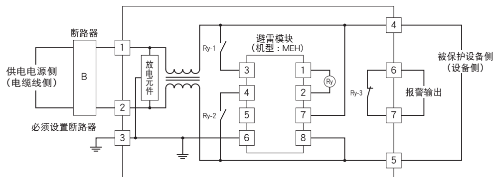
· 避雷模块 (机型: MEH) 简易电路图
